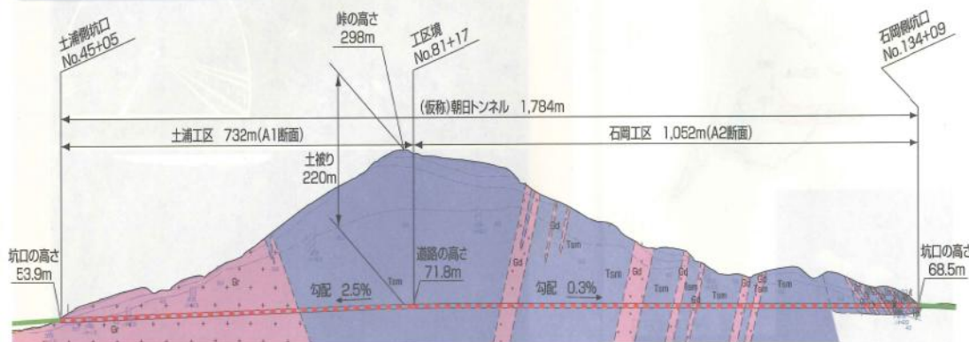
地質縦断面図
